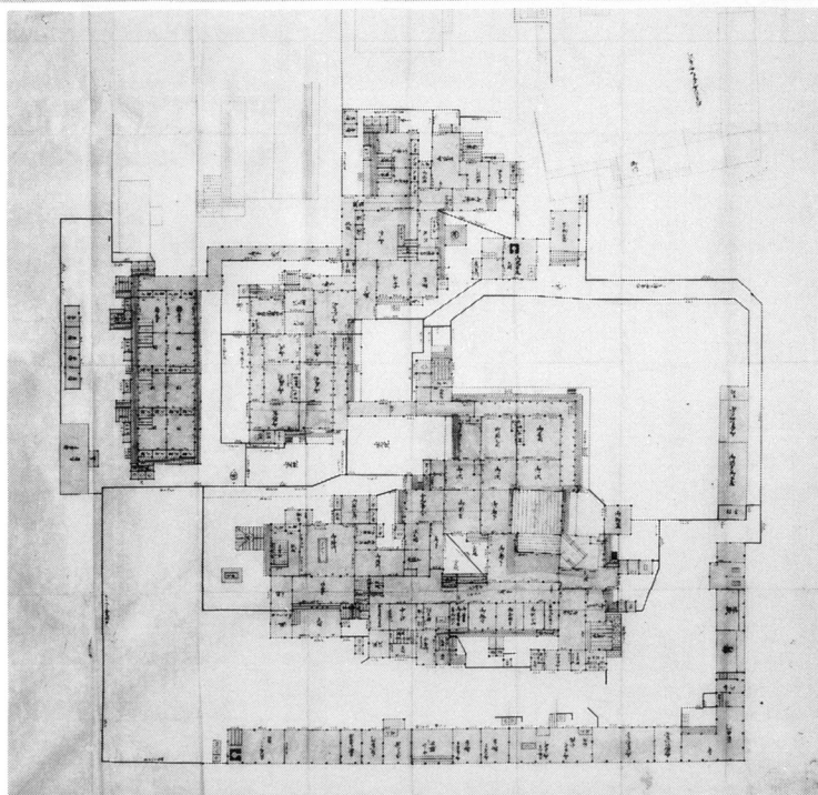
上：「祐仙院様御居宅御絵図」（金沢市立図書館所蔵加越能文庫、特16.18—149）
